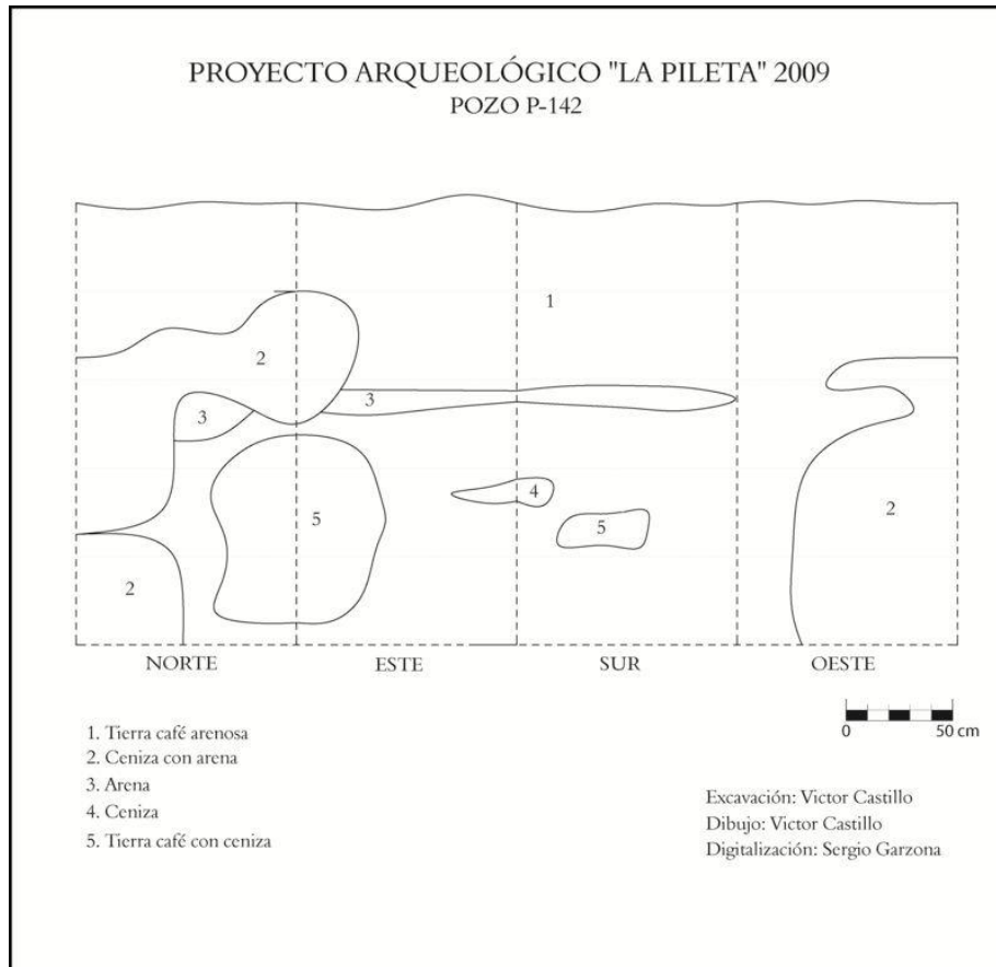
Figura 5 Perfil de la unidad P142 que ilustra la estratigrafía típica del basurero ubicado al este del terreno. Excavación y dibujo V. Castillo. Digitalización S. Garzona.
