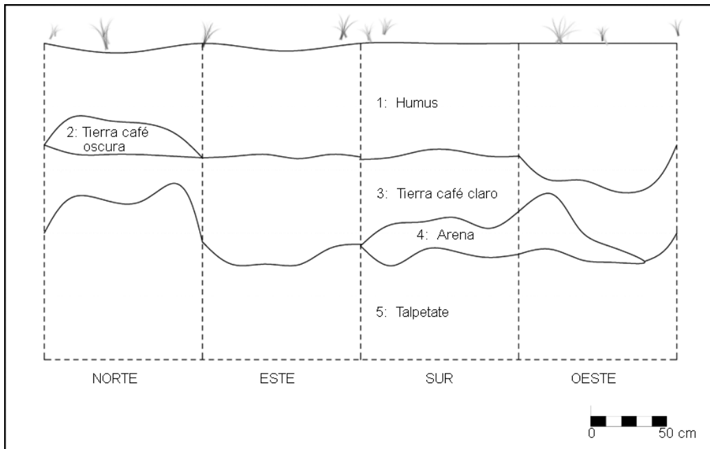
Figura 4 Perfil del pozo B17, que ilustra la estratigrafía típica del terreno. Proyecto Arqueológico "La Pileta" 2009. Excavación y dibujo G. Guerra. Digitalización S. Garzona.
