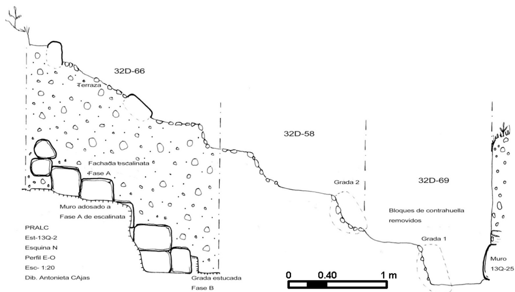
Fig.8: Perfil de la fachada norte de la gradería de Estra. 13Q-2 (dibujo por Antonieta Cajas).
