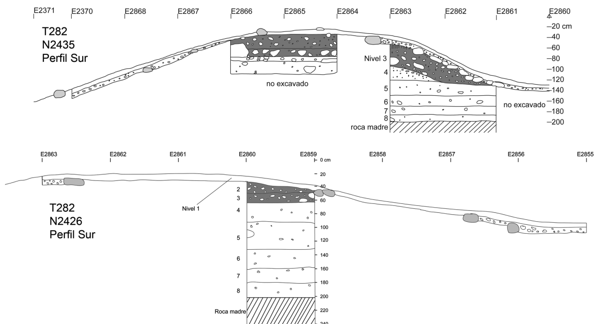
Fig.5: Perfiles de Estructura T282 de Tayasal mostrando la construcción del Clásico Terminal (gris oscuro) sobre la construcción del Preclásico Tardío (blanco): Estructura central T282 (arriba) y Estructura T282-2 (abajo).
