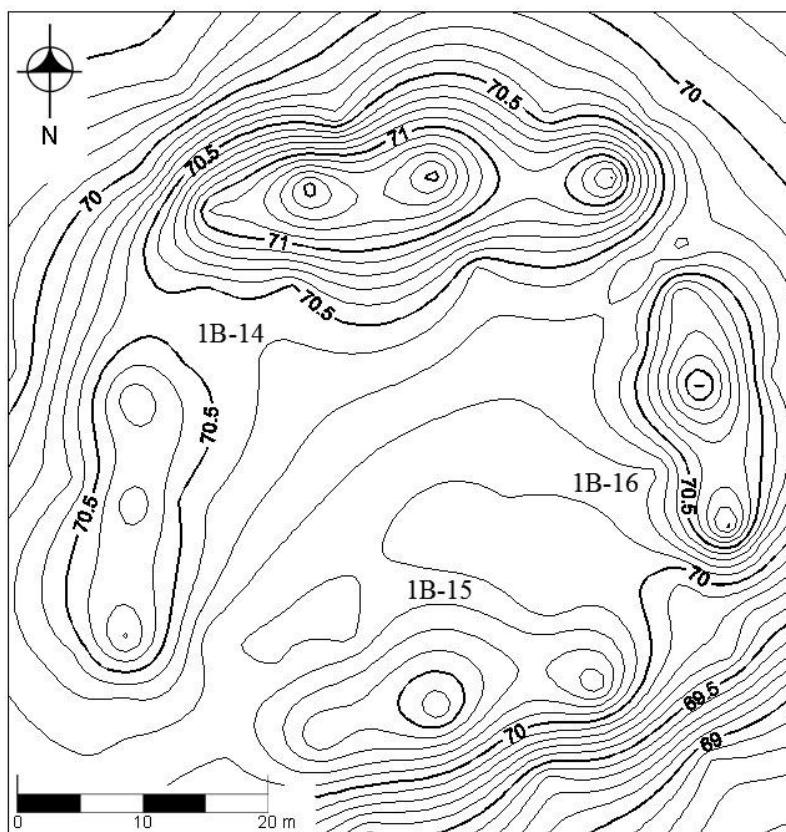
Figura 2 Plano topográfico del Grupo Este (Levantamiento J. Crasborn 2009).
