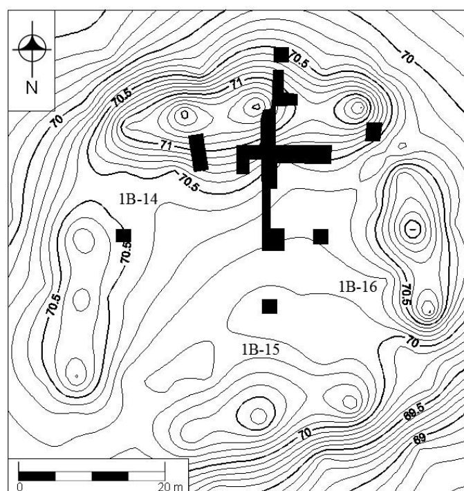
Figura 3 Plano topográfico del Grupo Este y planta de excavaciones (Levantamiento J. Crasborn 2009).
