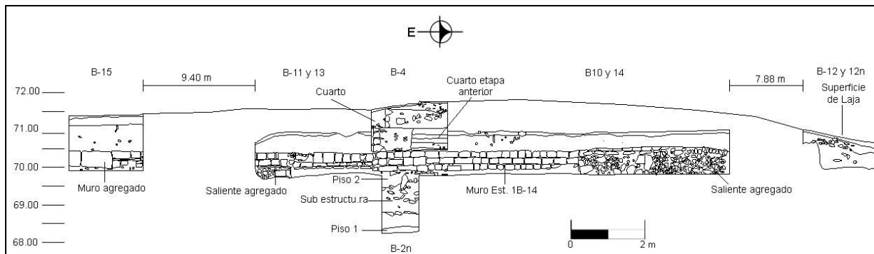
Figura 5 Corte Este-Oeste, Estructura 1B-14 (Dibujo E Marroquín, Calco J. Crasborn 2010).
