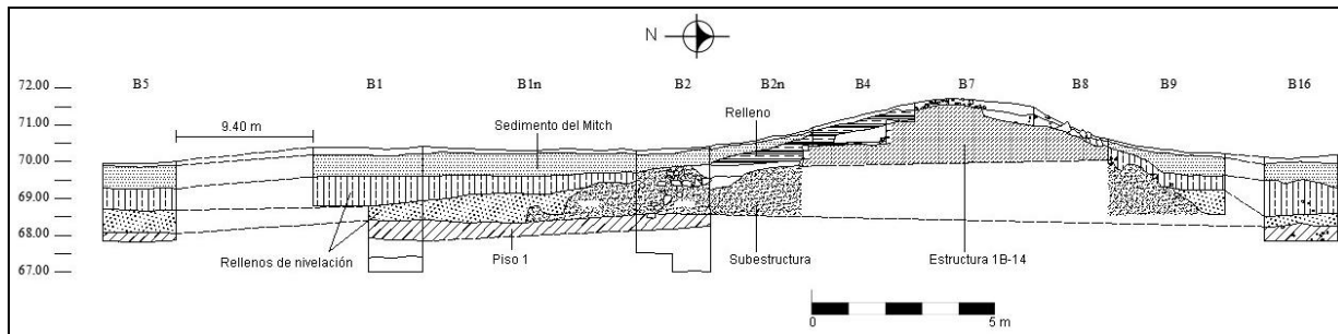
Figura 4 Corte Norte-Sur, Estructura 1B-14 (Dibujo E. Marroquín, Calco J. Crasborn 2010).
