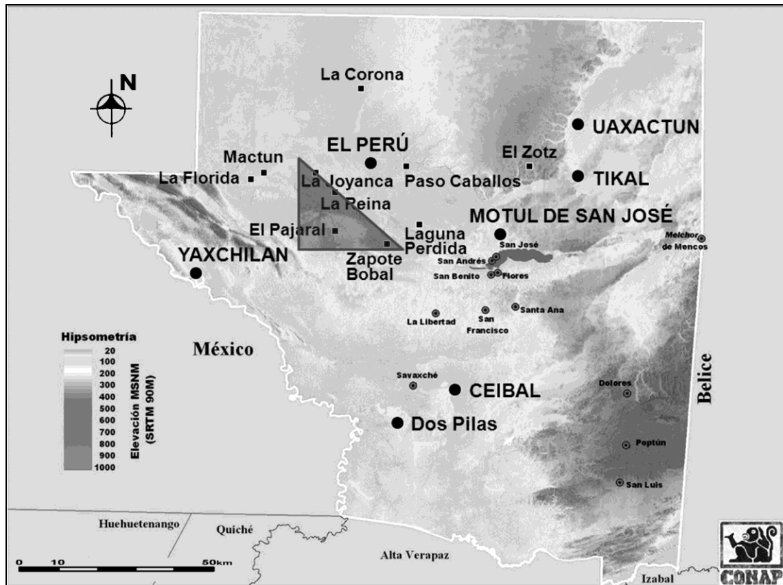
Figura 1. Mapa topográfico de Petén
