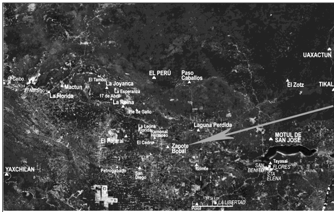
Figura 2. Mapa del oeste de Petén
