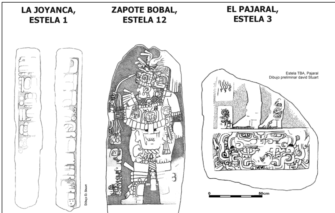
Figura 8. Ejemplos de monumentos de Hiix Witz
