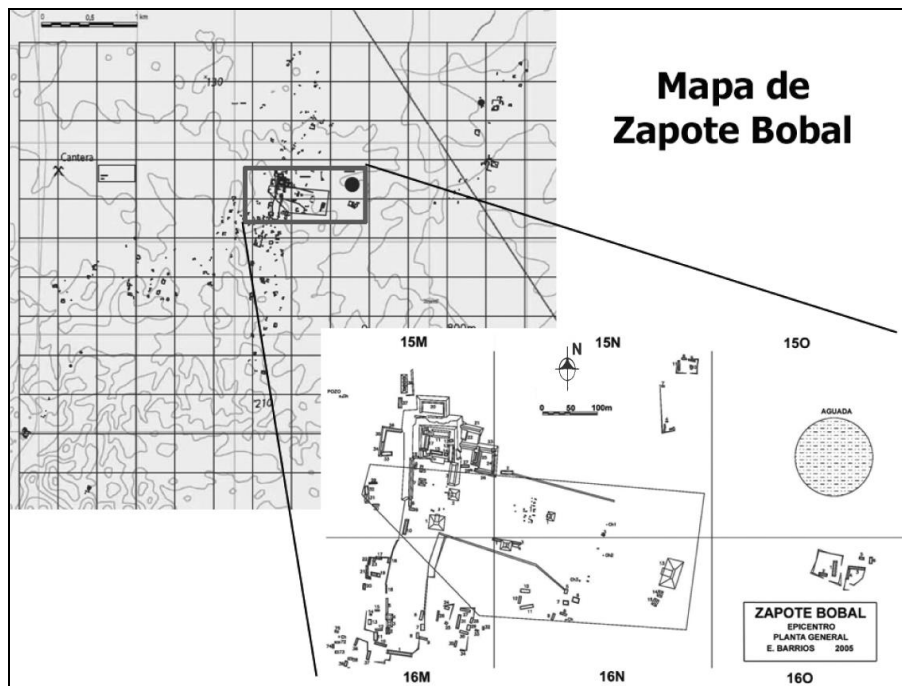
Figura 6. Mapa de Zapote Bobal
