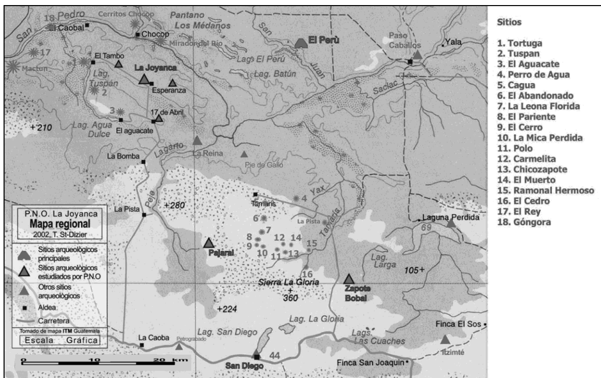
Figura 3. Mapa regional de Hiix Witz
