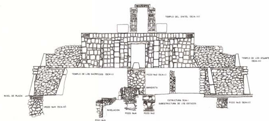
FIGURA No8— PERFIL OESTE DEL SISTEMA CONSTRUCTIVO (ESTRATIGRAFIA) DE LA ESTRUCTURA 5C4
