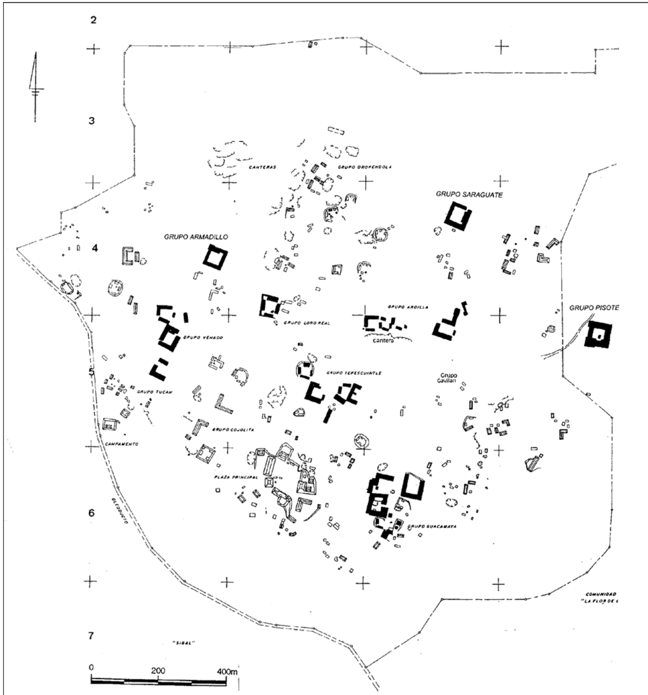
Figura 1 Plano preliminar del sitio La Joyanca (IDAEH, Basic Resources, 1996)
