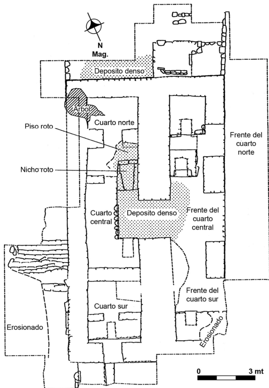
Figura 6 Planta de la Estructura M7-32
