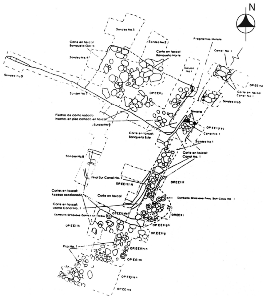
FIG. No. 474 PLANTA OP. EE I I J "CASA EL ESCONDITE" PROYECTO NACIONAL ABAJ TAKALIK 1997 MINISTERIO DE CULTURA Y DEPORTES / IDAEH RESPONSABLE: LICDA. CHRISTA SCHIEBER DE LAVARRADA LEVANTADO: MARIO TOMÁS DE LEÓN, JUAN LIMA CALCO: MARIO TOMÁS DE LEÓN
