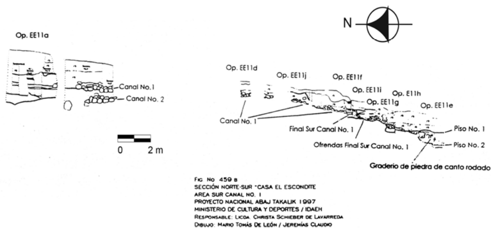
Figura 6 B Sección norte-sur de El Escondite, Area Sur, Canal 1 (Dibujo: Mario Tomás De León y Jeremías Claudio)
