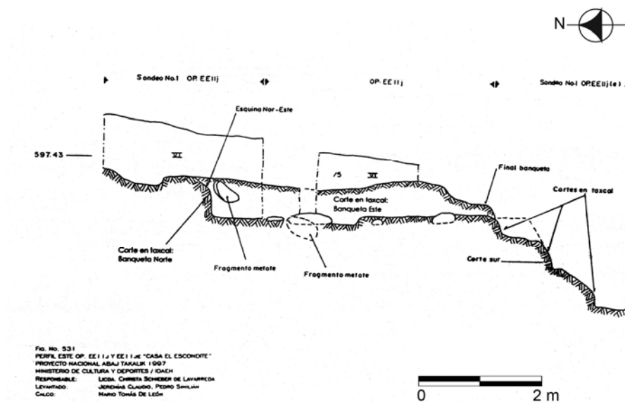
Figura 14 Perfil este, Casa El Escondite (Levantado: Jeremías Claudio y Pedro Similián; calco: Mario Tomás De León)
