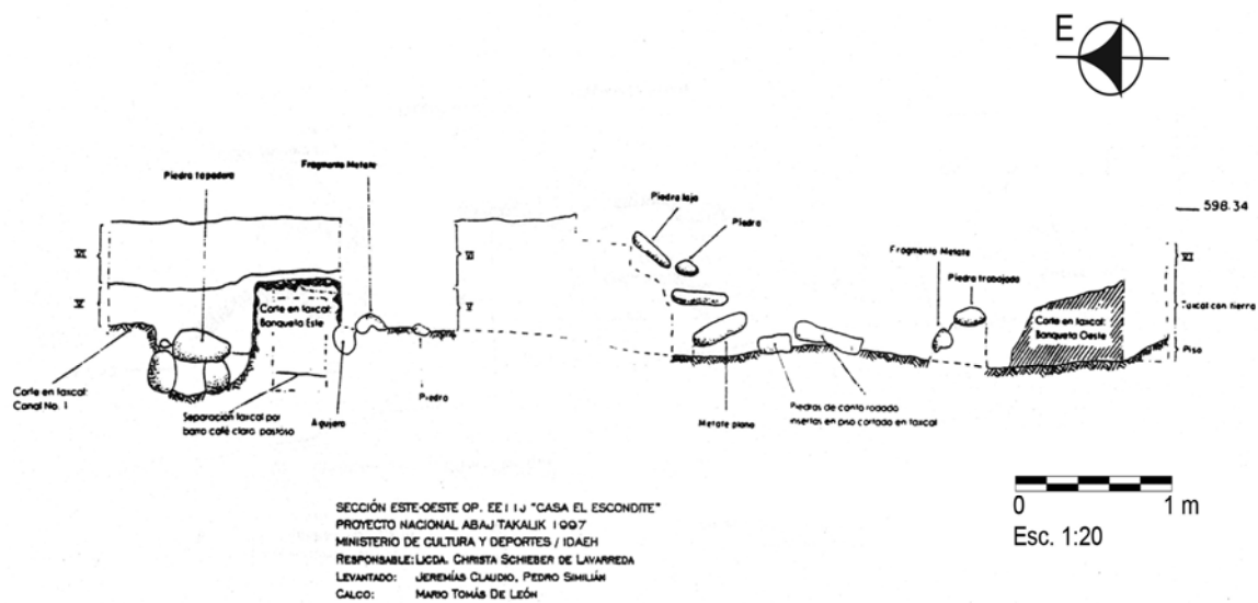
Figura 13 Sección este-oeste, Casa El Escondite (Levantado: Jeremías Claudio y Pedro Similián; calco: Mario Tomás De León)
