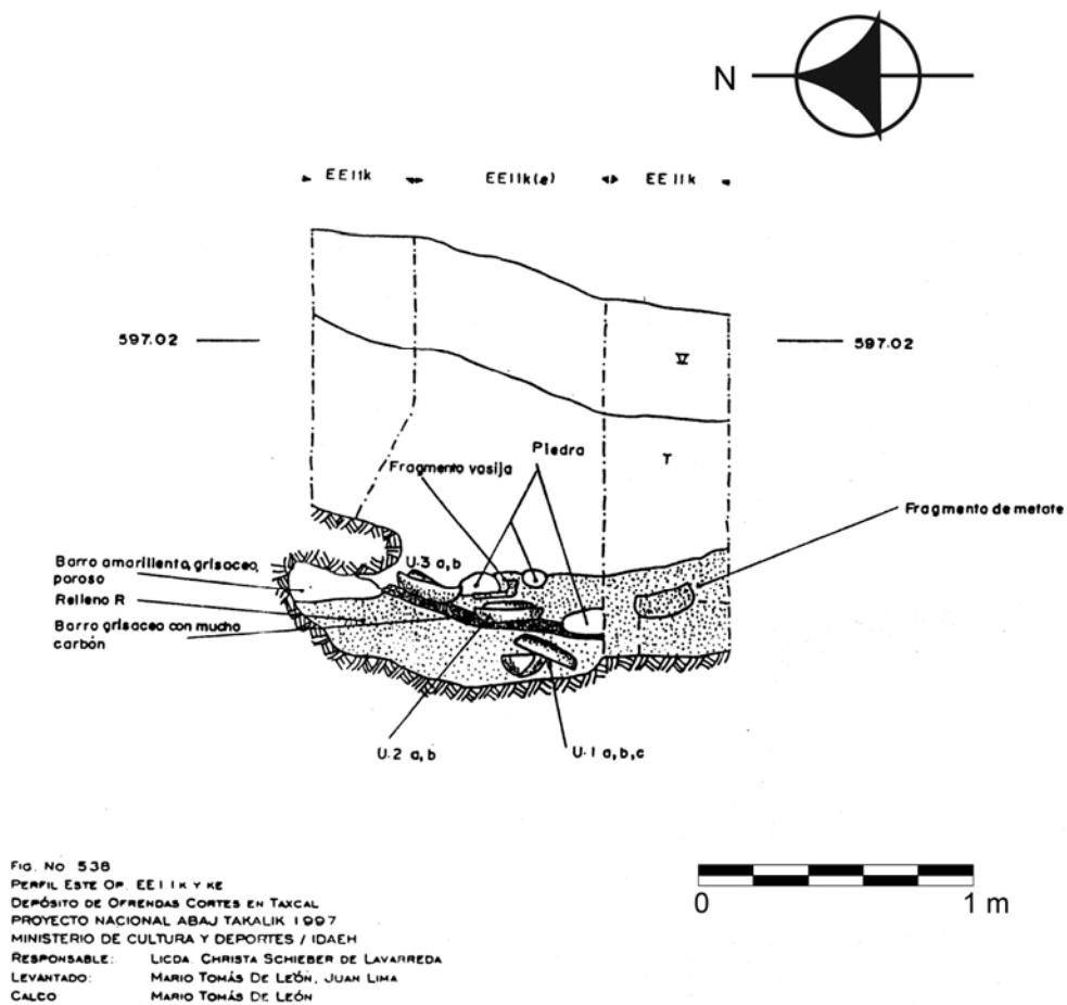
Figura 10 Perfil este del Depósito de Ofrendas, Cortes En taxcal (Levantado: Jeremías Claudio y Juan Lima; calco: Mario Tomás De León)
