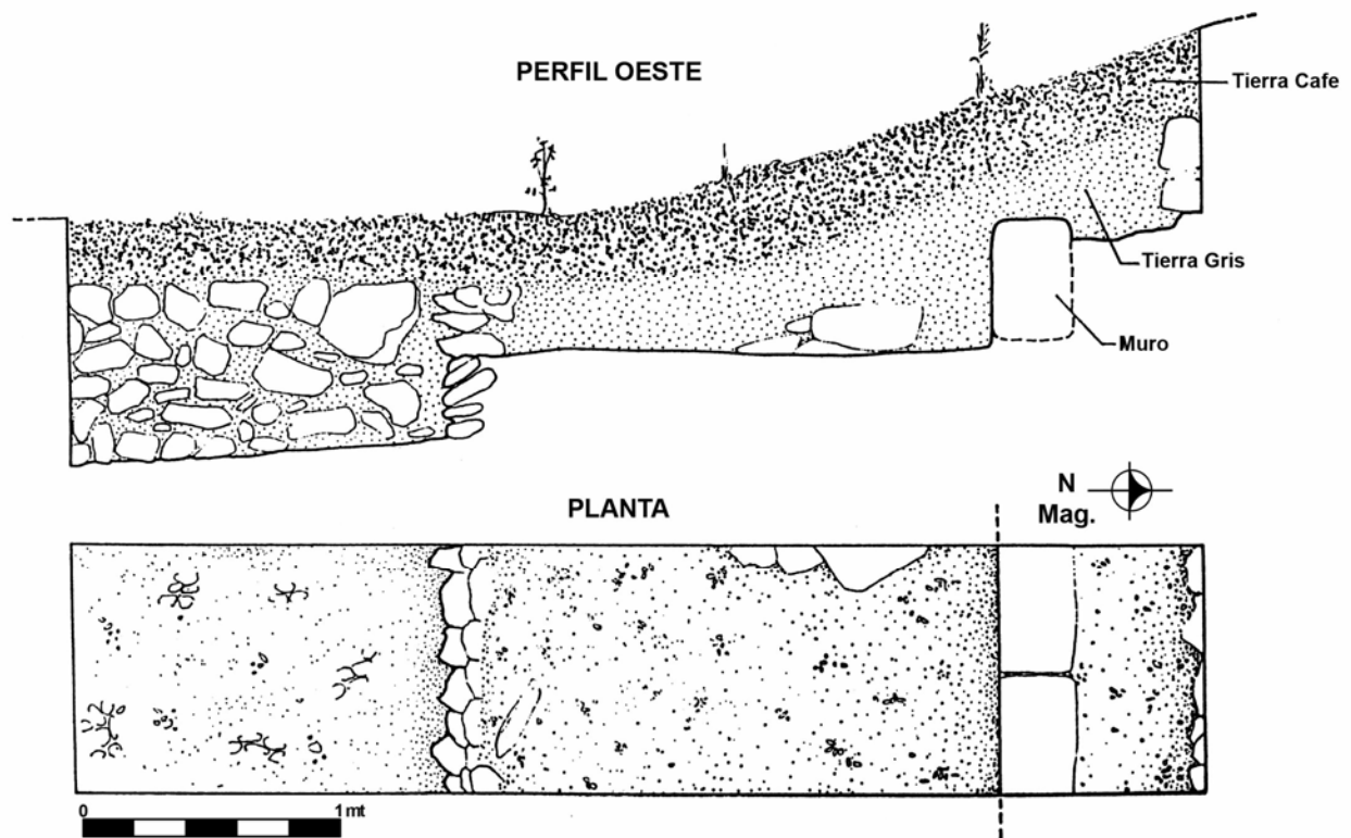
Figura 9 Planta de la Operación 30A, indicando el muro basal del edificio
